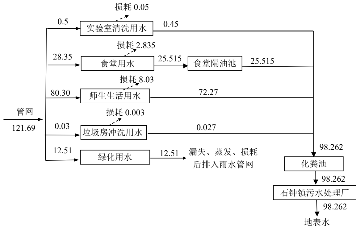
图 3-1 项目水平衡分析图 单位：m³/d
