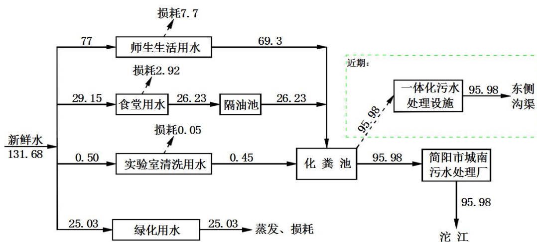
图 3-1 项目水平衡分析图 单位：m 3 /d
