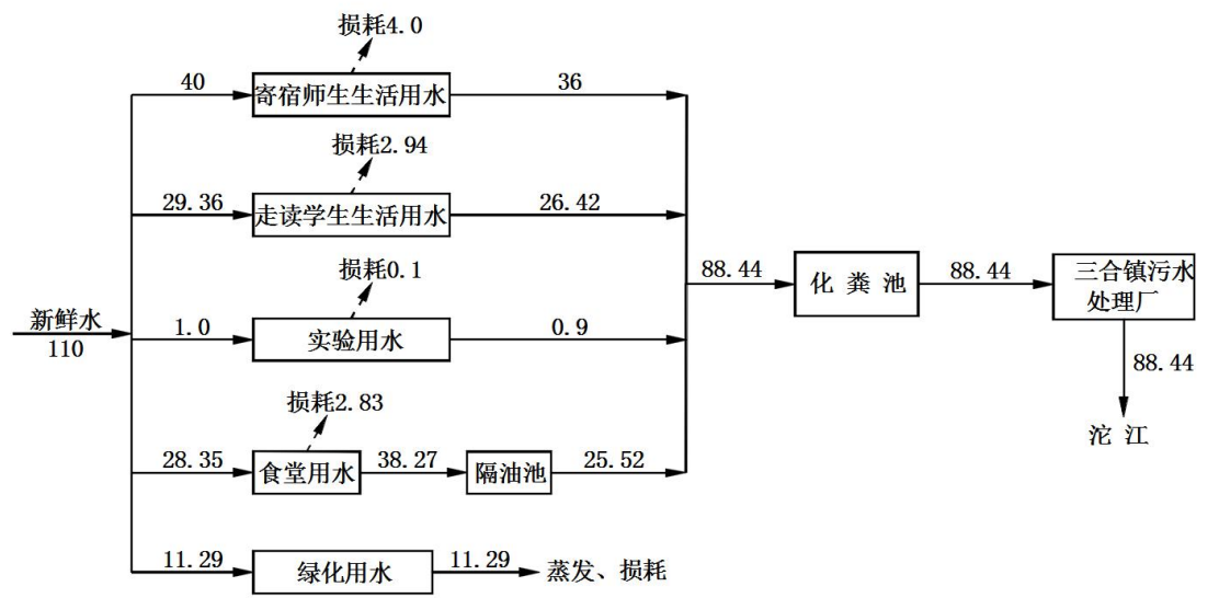
图 3-1 项目水平衡分析图 单位：m 3 /d
