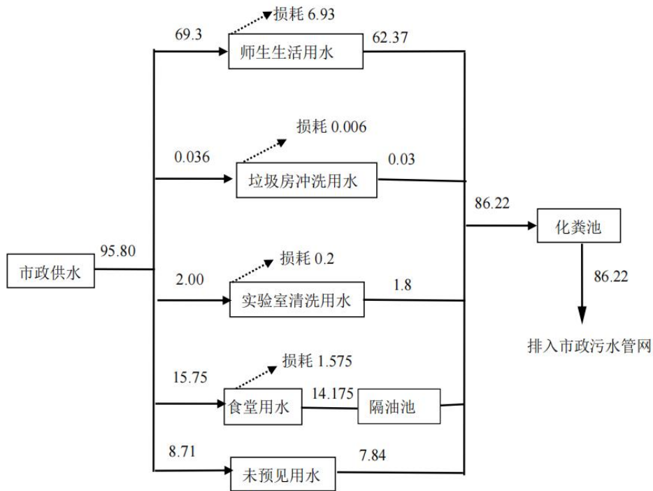
图 3-1 项目水平衡分析图 单位：m 3 /d
