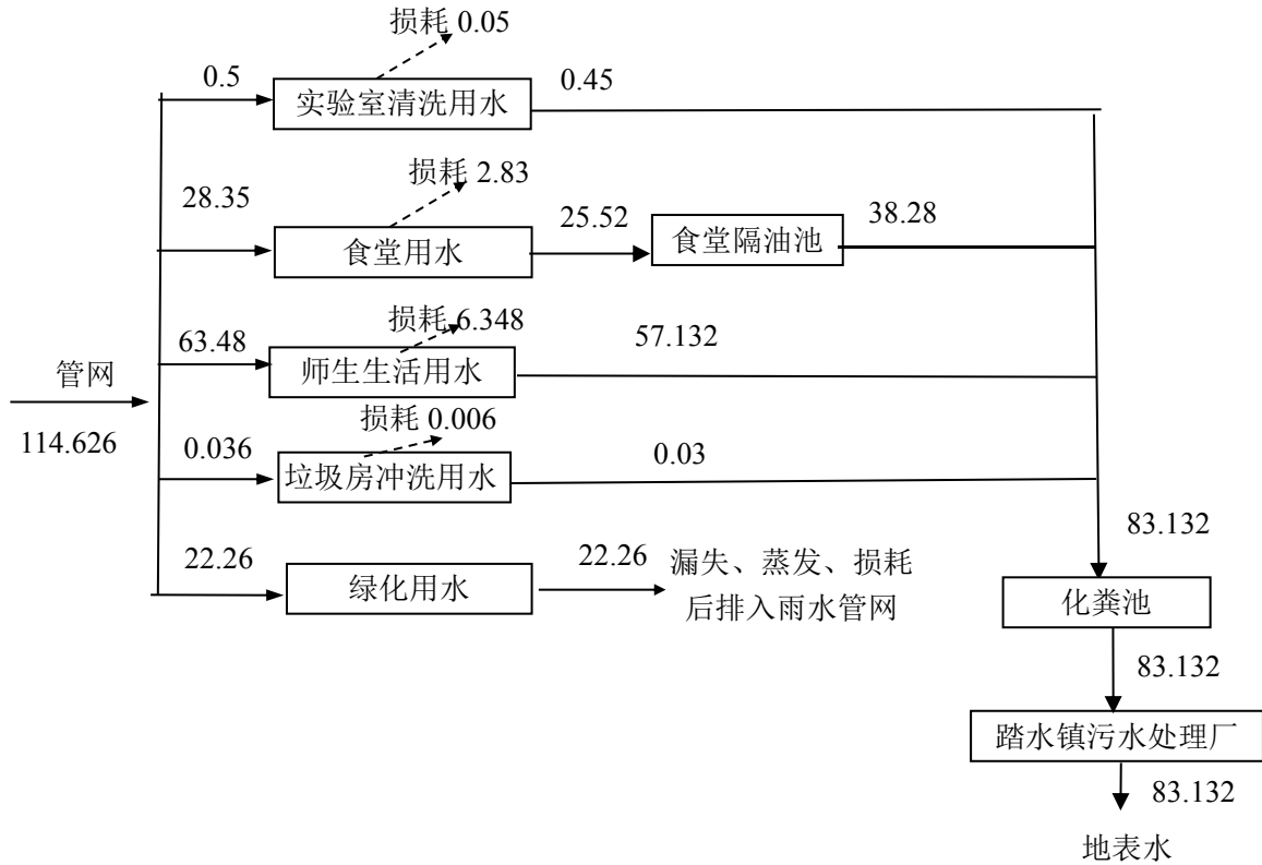
图 3-1 项目水平衡分析图 单位：m 3 /d
