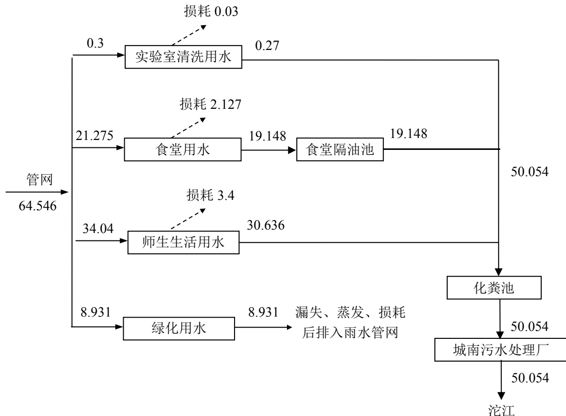
图 3-1 项目水平衡分析图 单位： \text{m}^3/\text{d}
