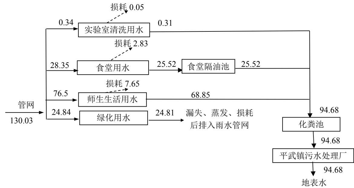
图 3-1 项目水平衡分析图 单位：m³/d
