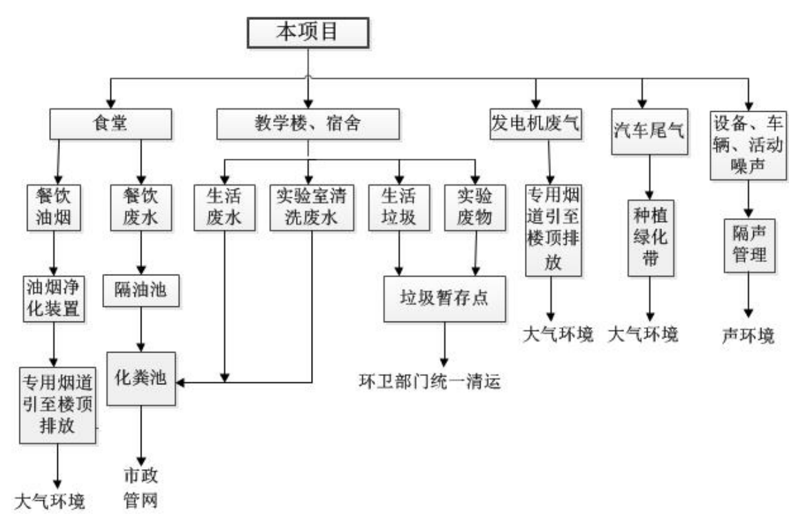
图 3-2 运营期工艺流程及产污环节位置图
