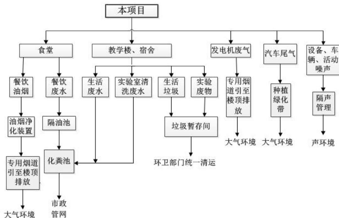
图 3-2 运营期工艺流程及产污环节位置图
