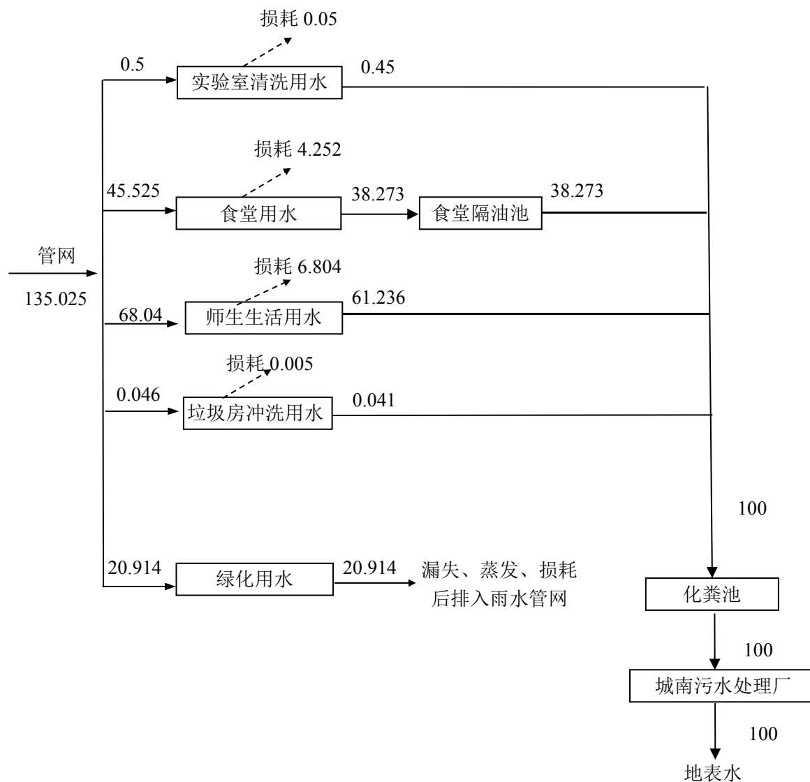
图 3-1 项目水平衡分析图 单位：m³/d
