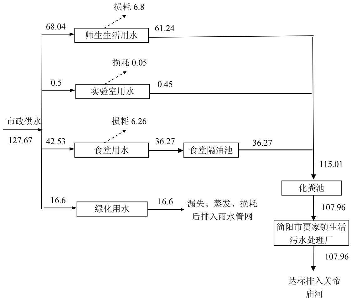
图 3-1 项目水平衡分析图 单位：m 3 /d
