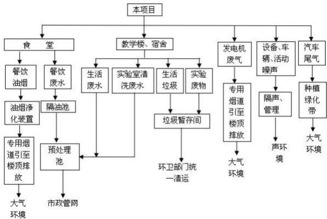
图 3-2 运营期工艺流程及产污环节位置图
