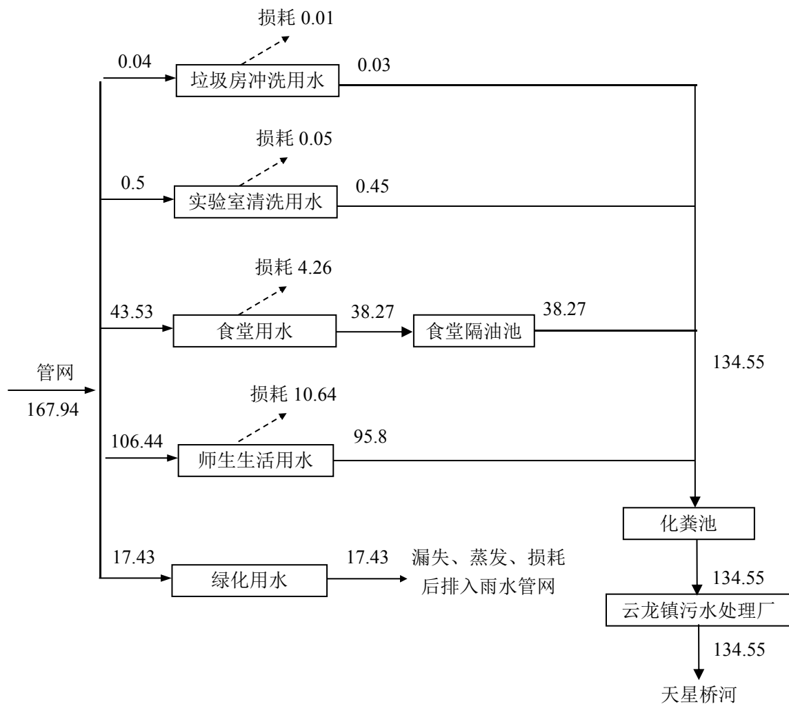
图 3-1 项目水平衡分析图 单位：m 3 /d
