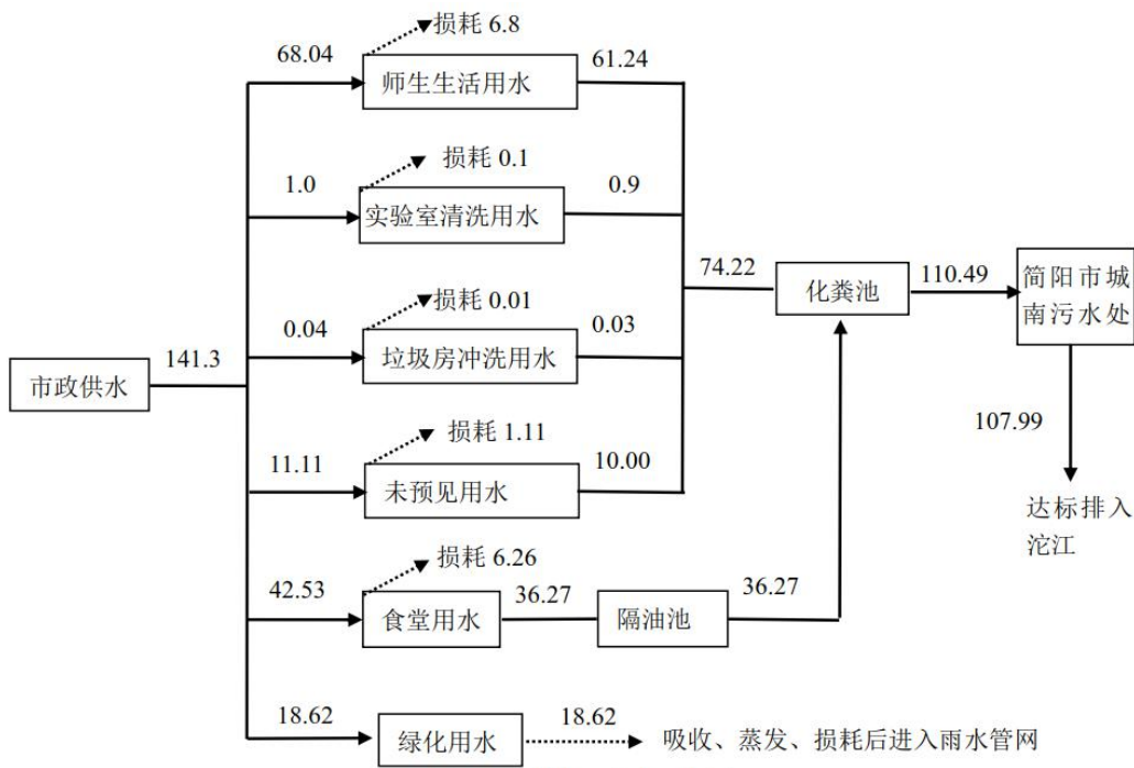
图 3-1 项目水平衡分析图 单位：m³/d
