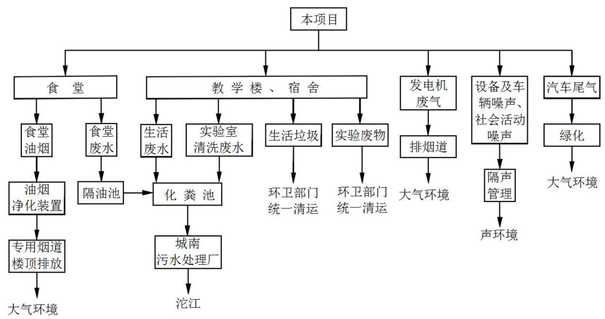
图 3-2 运营期工艺流程及产污环节位置图
