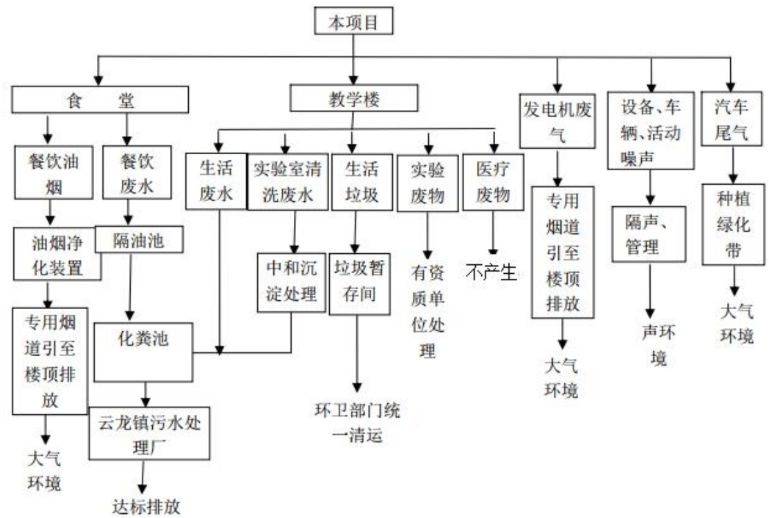
图 3-5 运营期工艺流程及产污环节位置图
