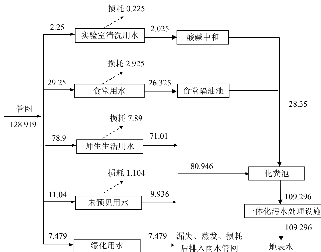
图 3-1 项目水平衡分析图 单位：m 3 /d
