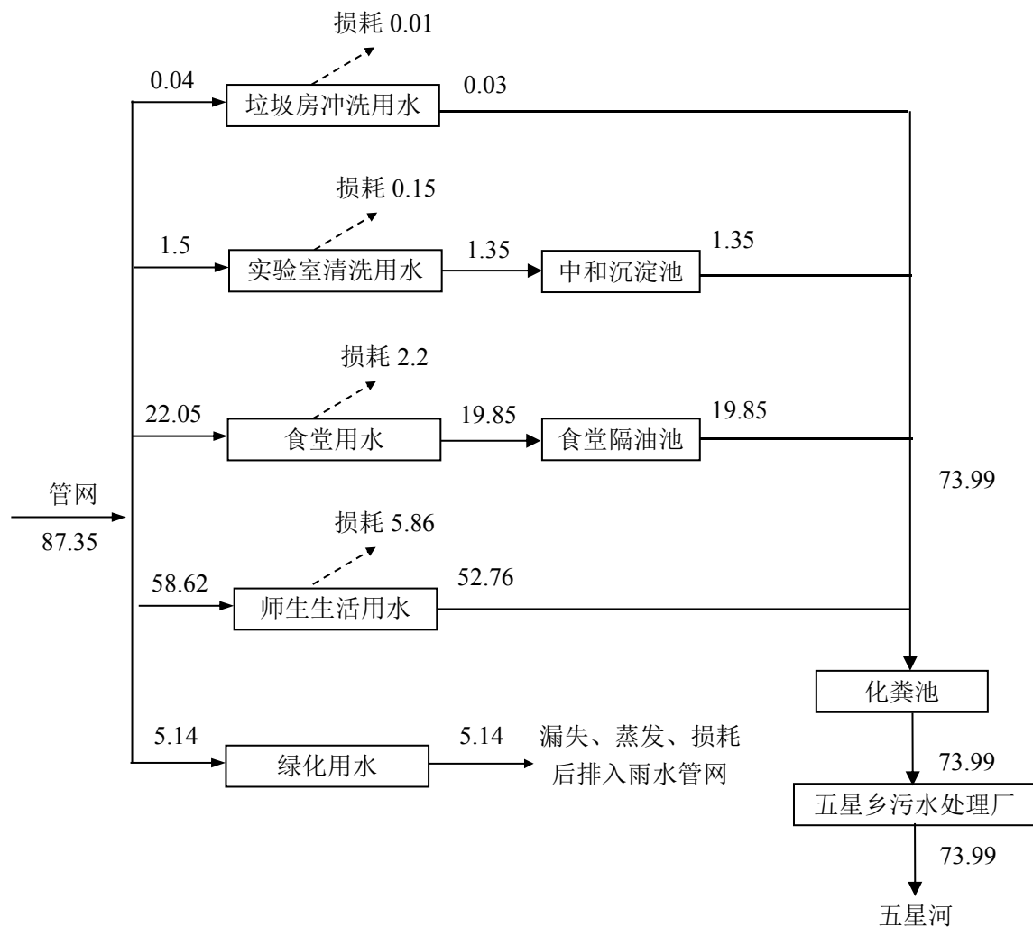
图 3-1 项目水平衡分析图 单位： \text{m}^3/\text{d}
