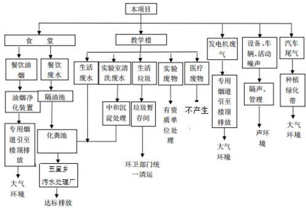
图 3-2 运营期工艺流程及产污环节位置图
