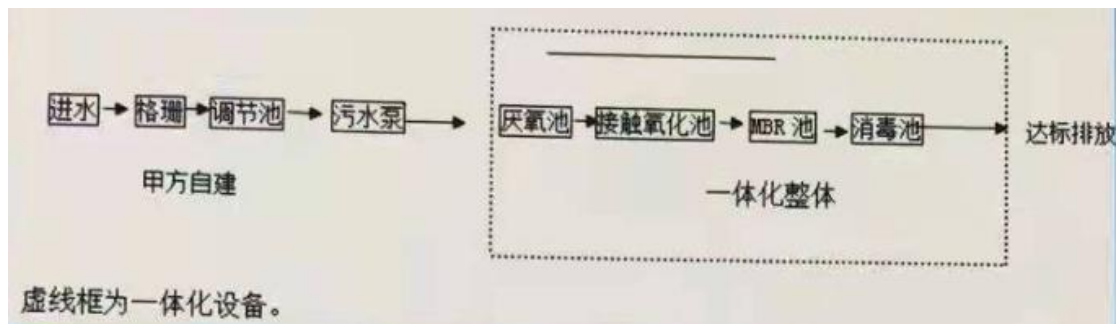
图 3-3 污水处理工艺流程图
