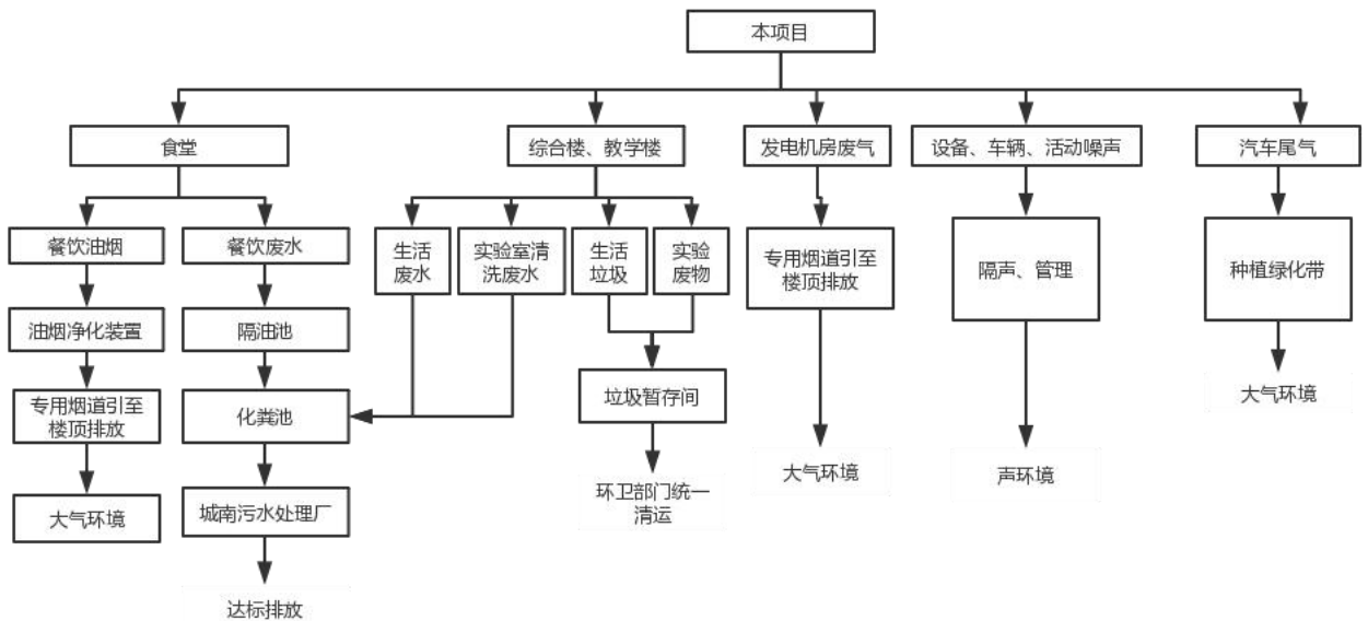
图 3-2 运营期工艺流程及产污环节位置图
