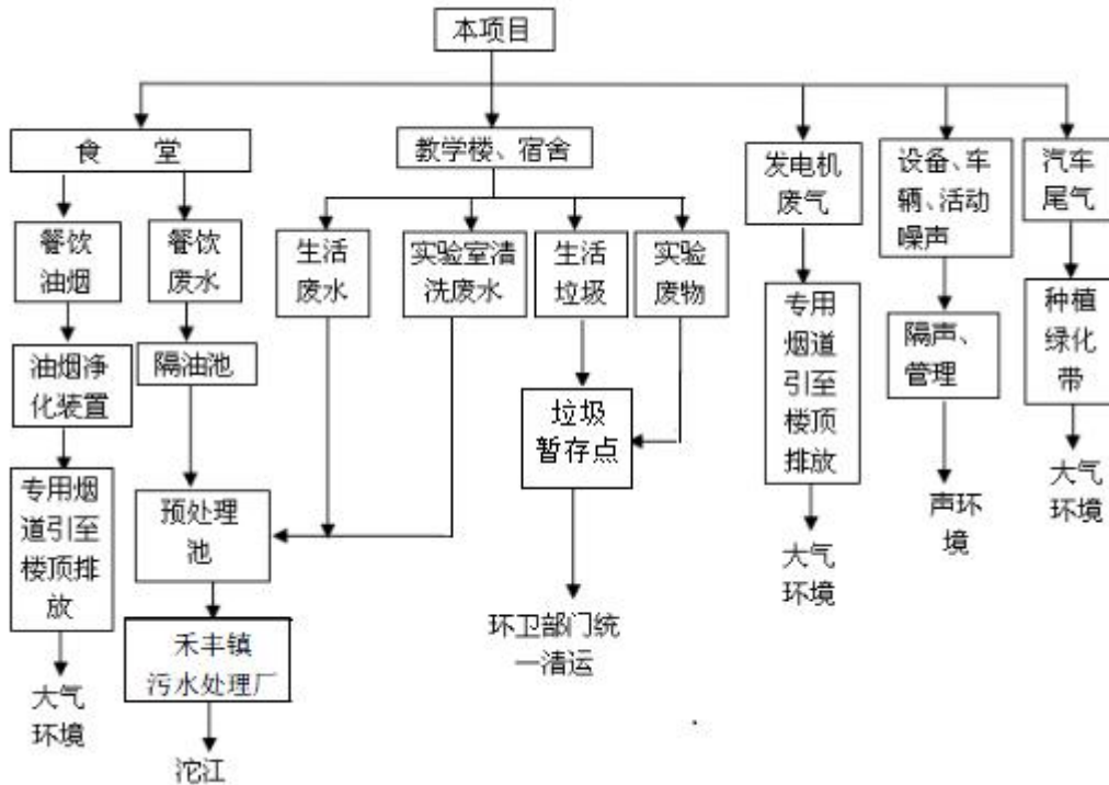
图 3-2 运营期工艺流程及产污环节位置图
