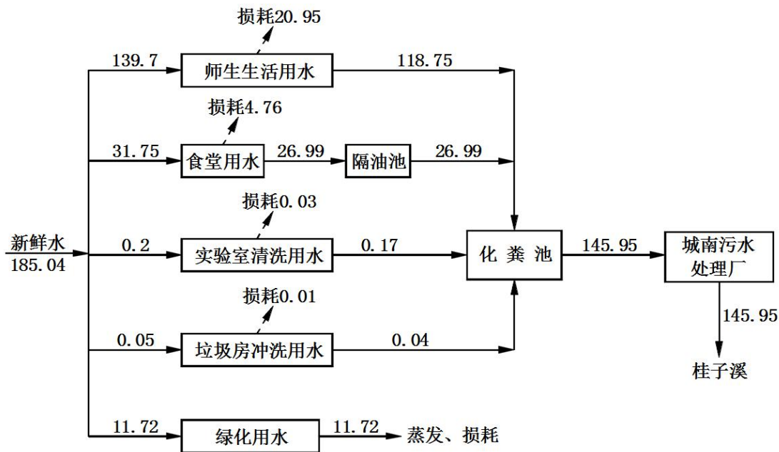
图 3-1 项目水平衡分析图 单位: m³/d
