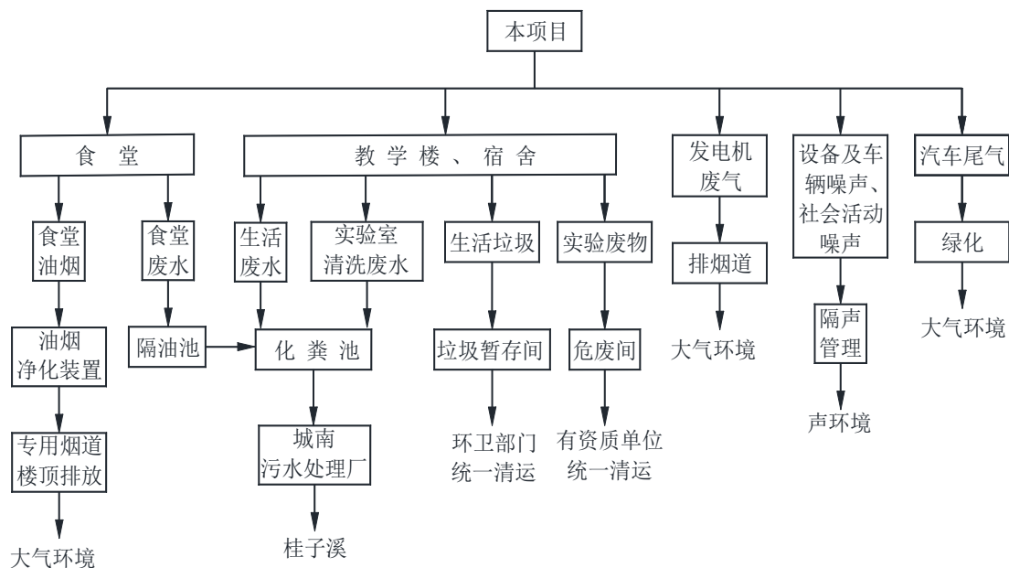
图 3-2 运营期工艺流程及产污环节位置图
