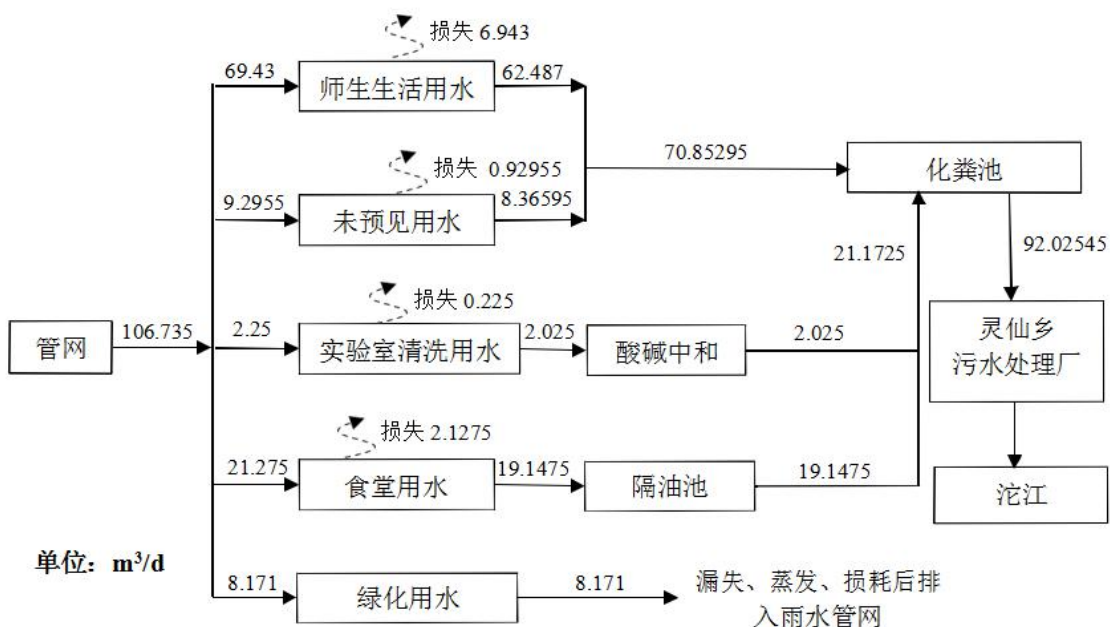
图 3-1 项目水平衡图单位: m 3 /d
