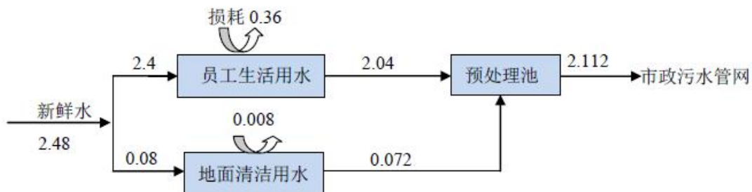
图 3-1 项目水平衡分析图 单位: m 3 /d
