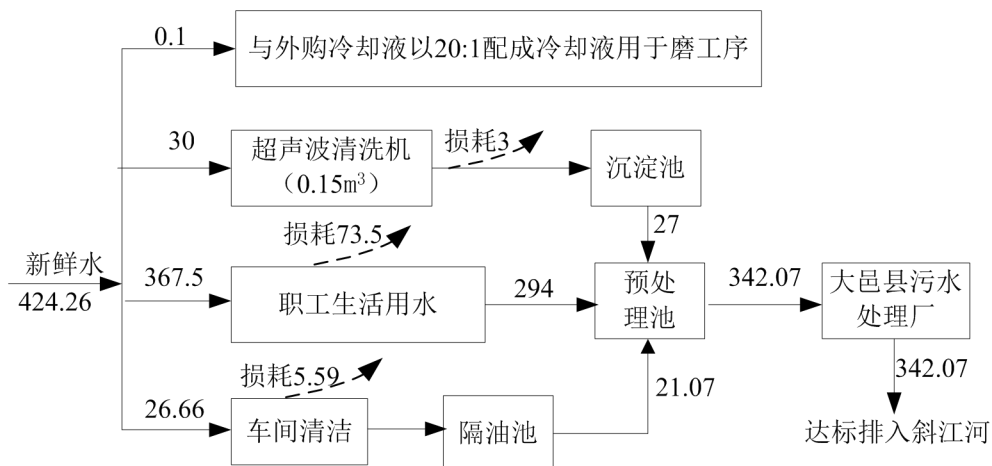
图 3-1 项目水平衡分析图 单位: m 3 /d
